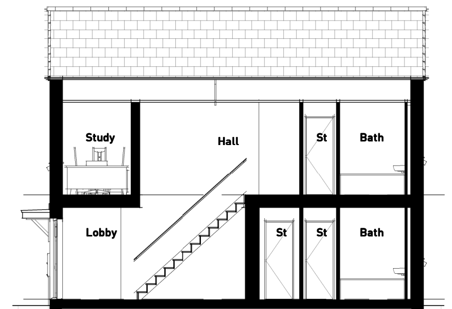
Section 1 : 100
